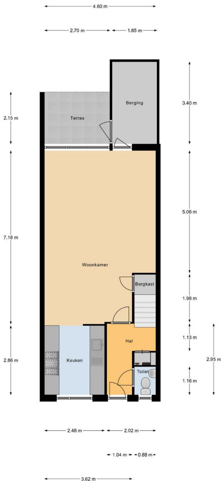
Begane Grond
