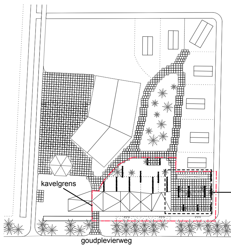
Situatie 1:2000
