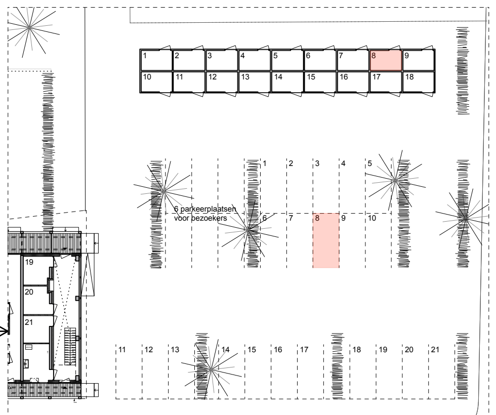
Bergingen + Hal+ Parkeren 1:350
