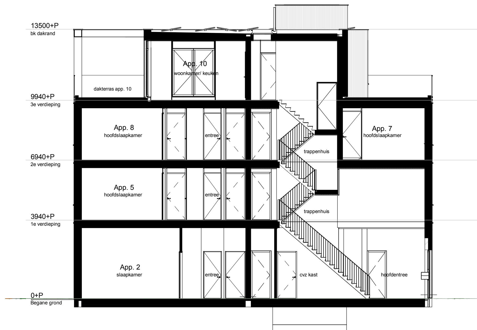
Doorsnede A-A
