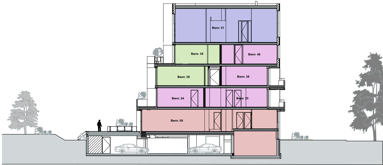
Doorsnede C
