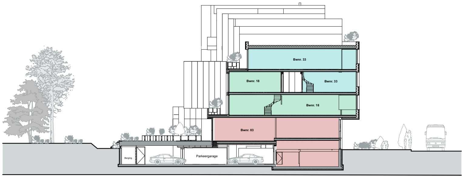
Doorsnede B
