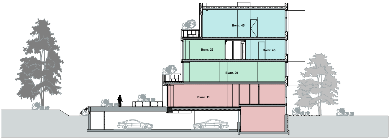
Doorsnede D
