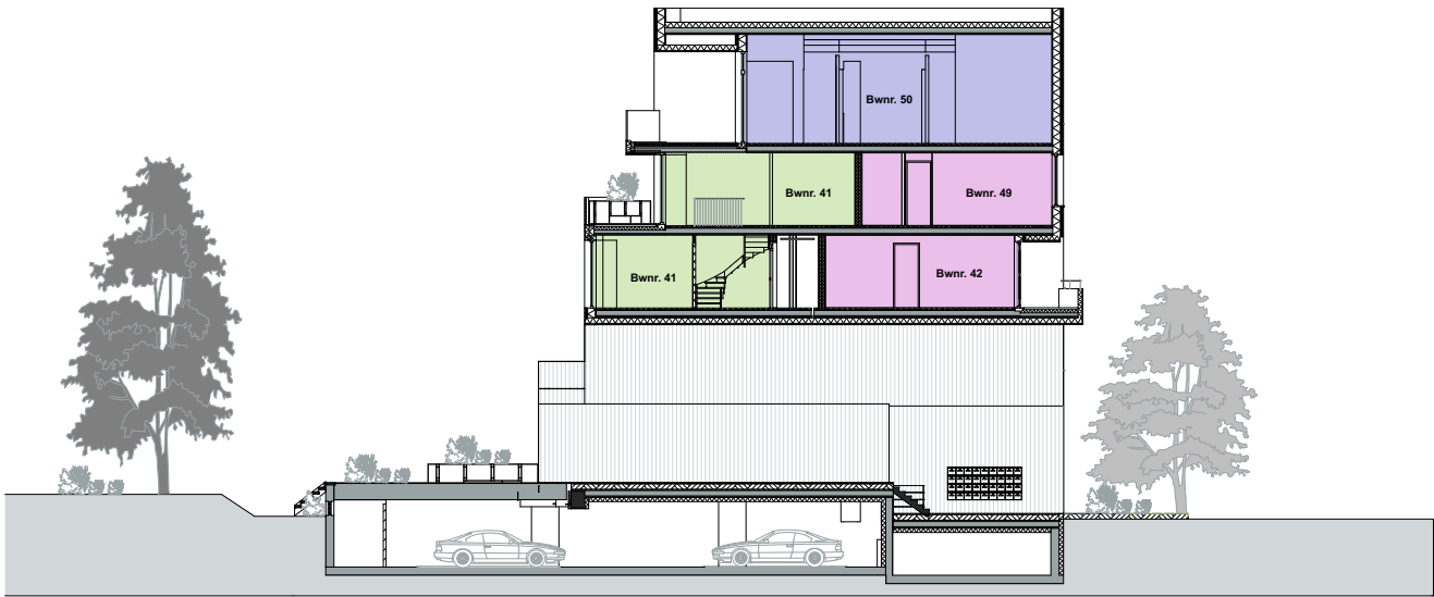
Doorsnede E
