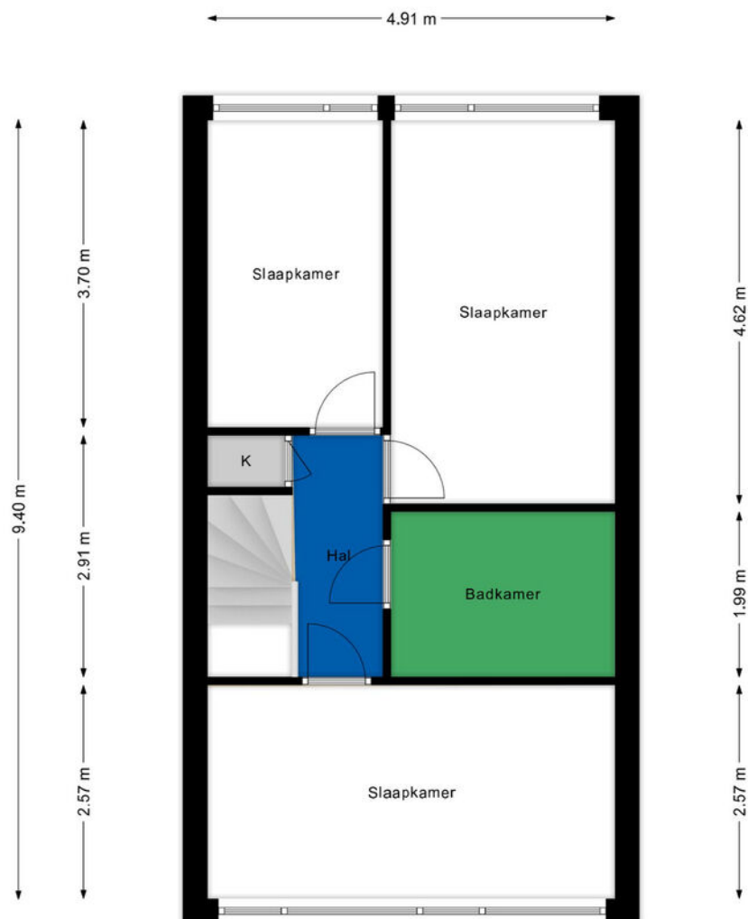
1e Verdieping
