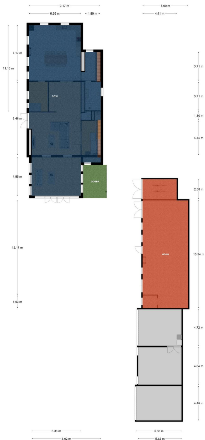
Begane Grond
