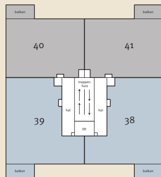
2e verdieping
