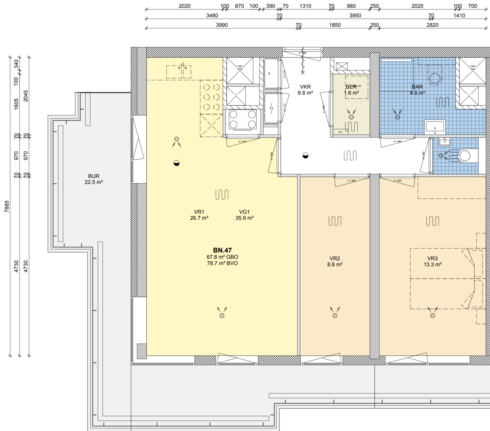
5e verdieping
