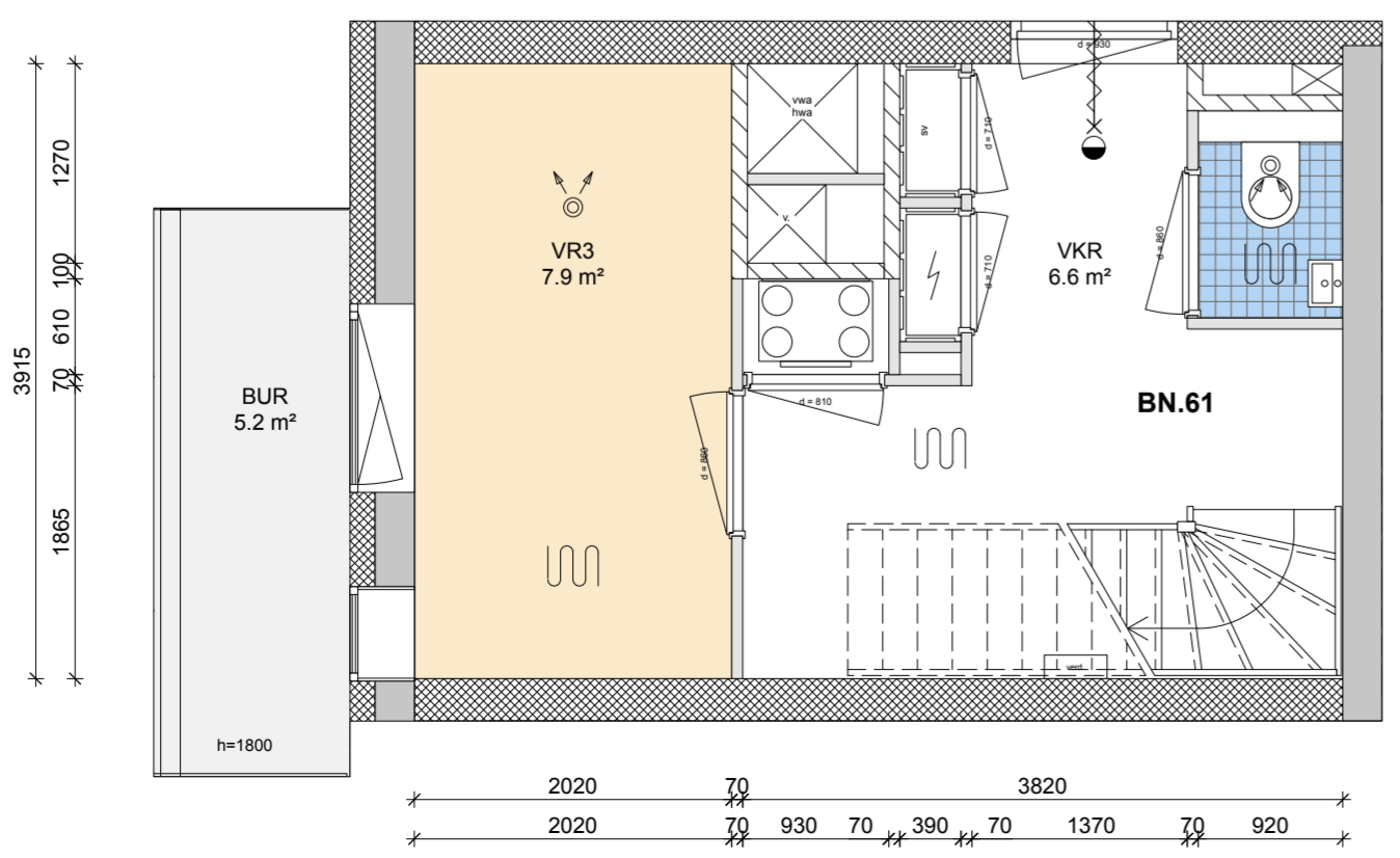
8e verdieping
