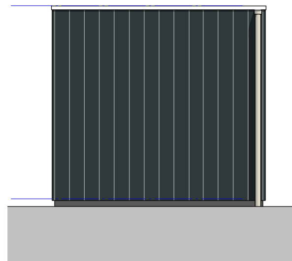
rechtergevel
