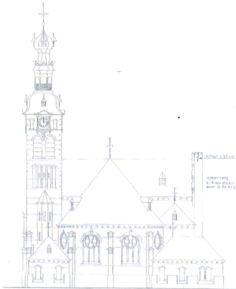
West gevel.
